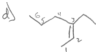
3-ethyl-2-hexene
